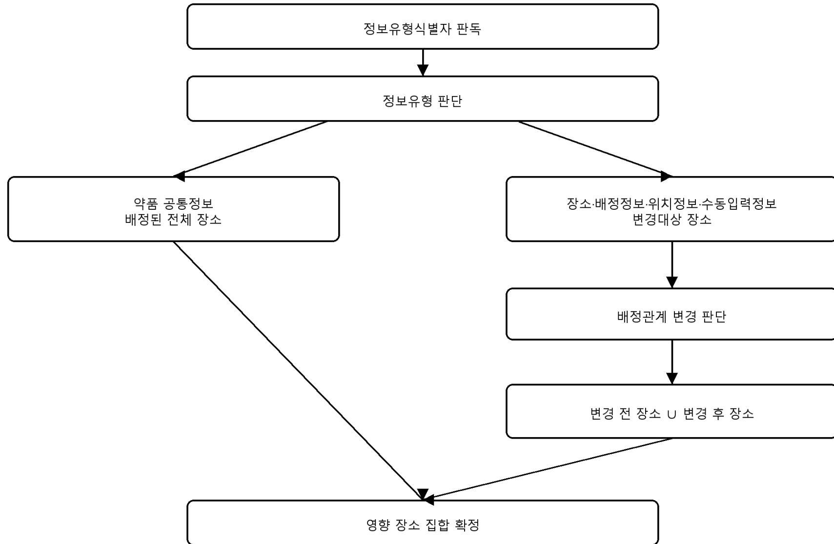
도 4. 영향 장소 집합 산출 흐름도
