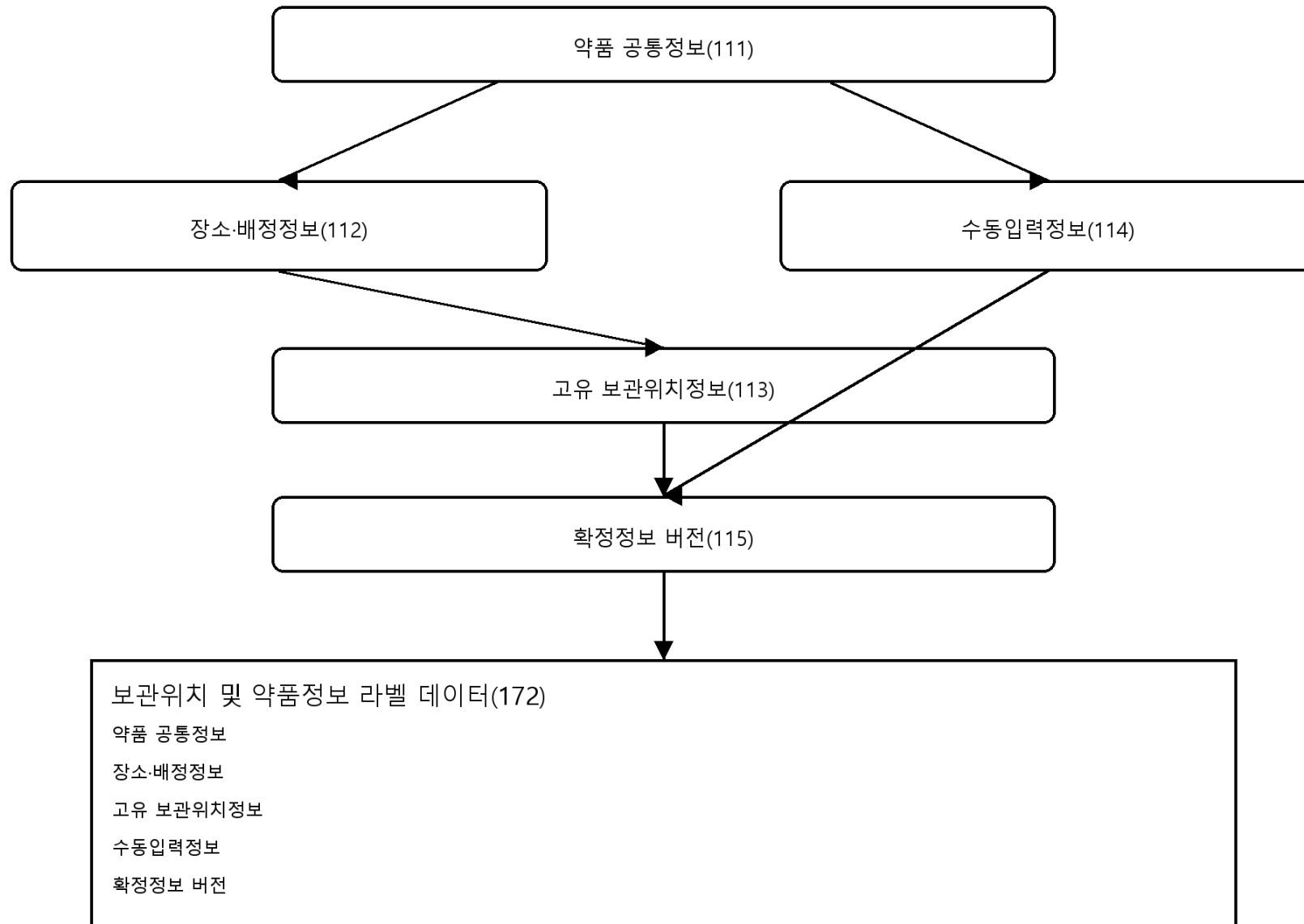
도 2. 데이터 구조도
