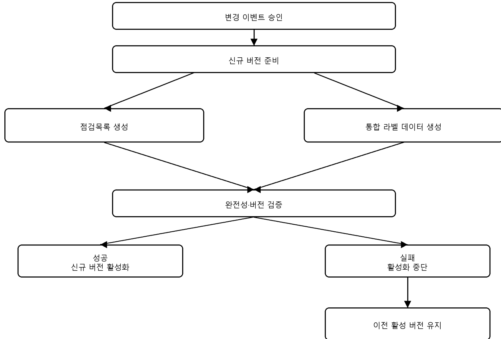
도 6. 버전 활성화 상태도
