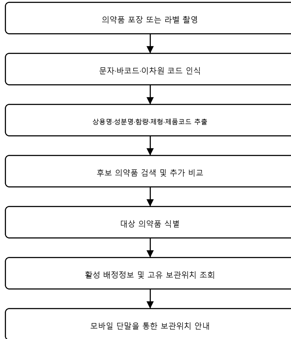
도 8. 카메라 인식 및 위치 안내 흐름도
