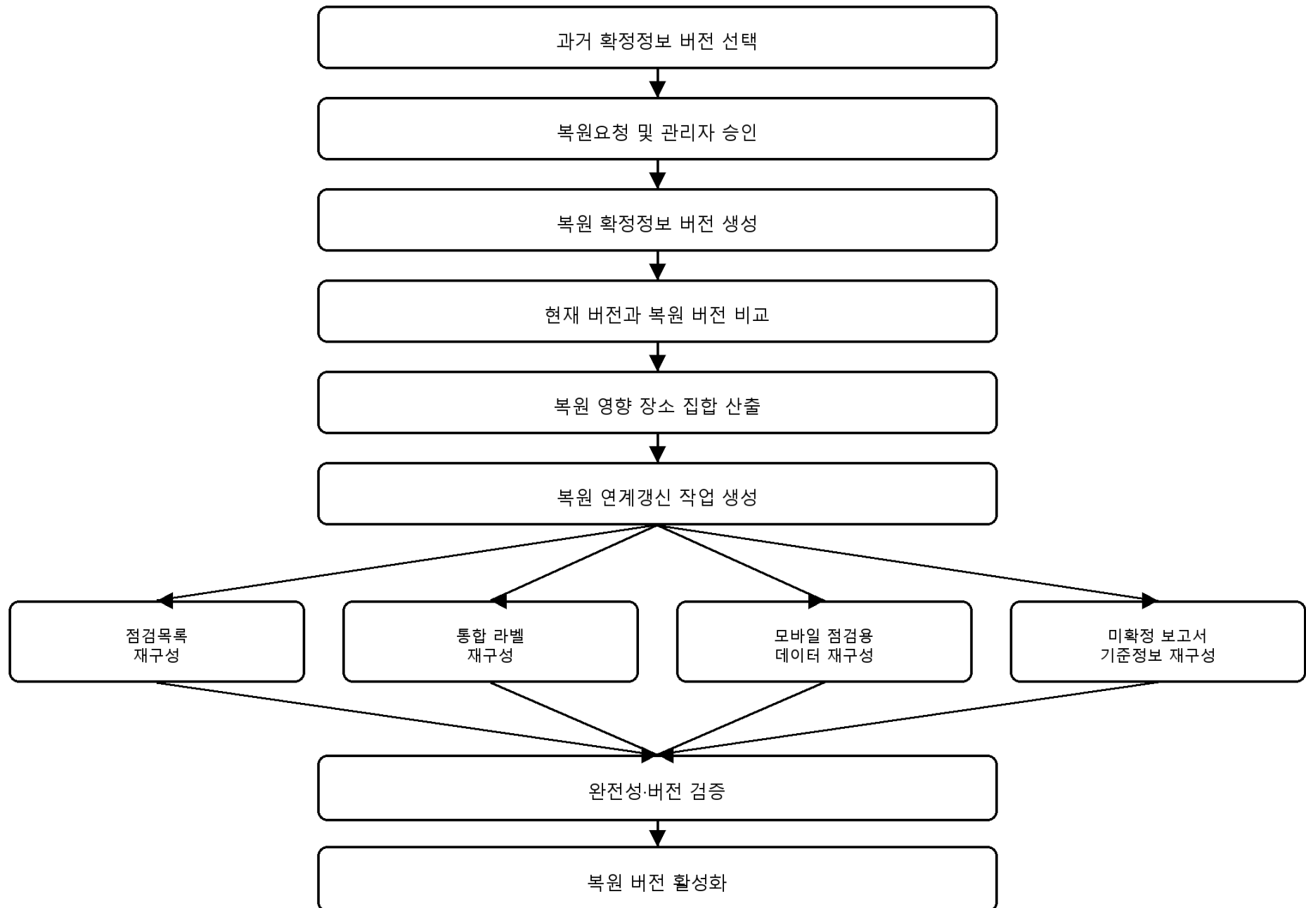
도 10. 과거 버전 복원 흐름도
