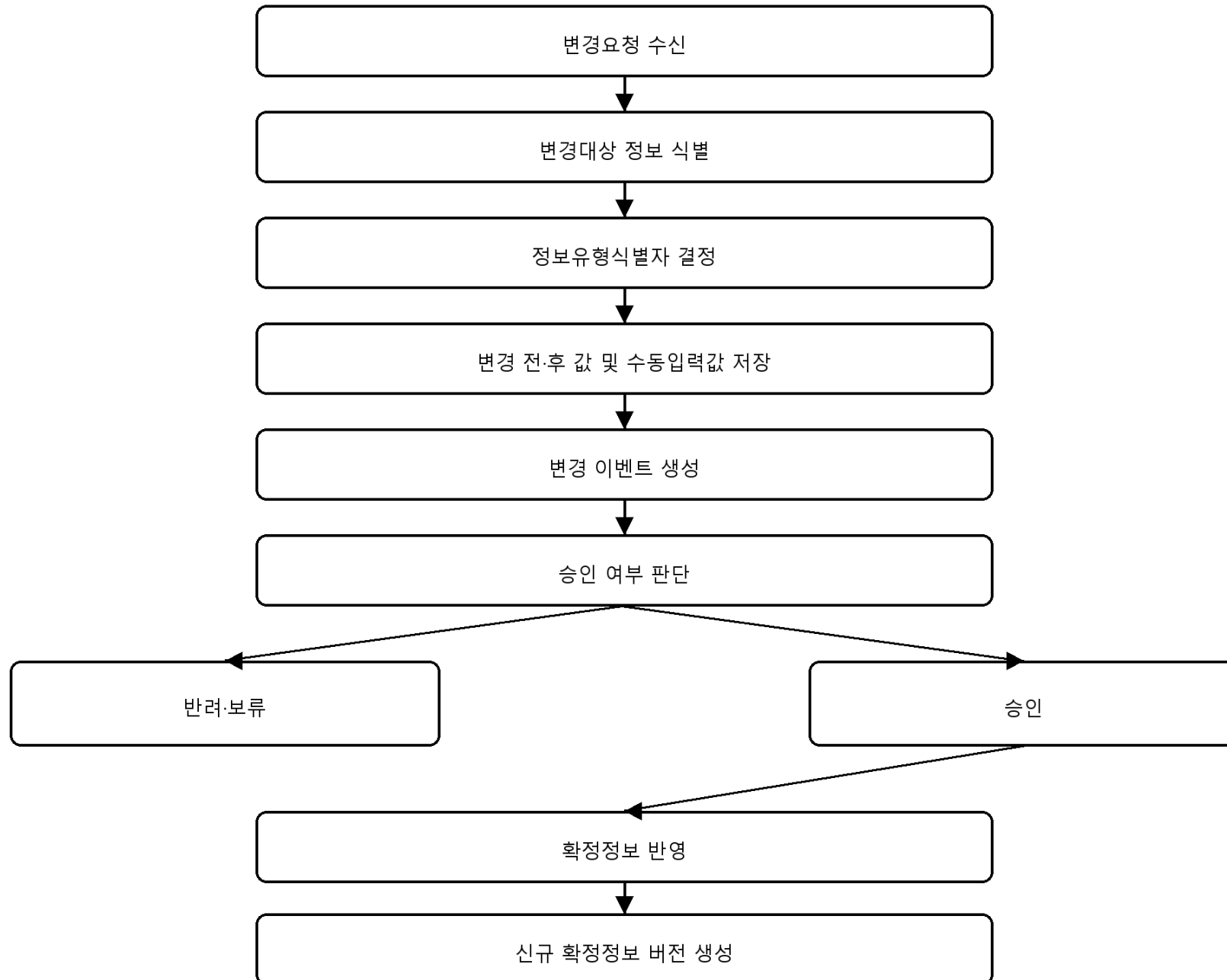
도 3. 변경 이벤트 및 버전 생성 흐름도
