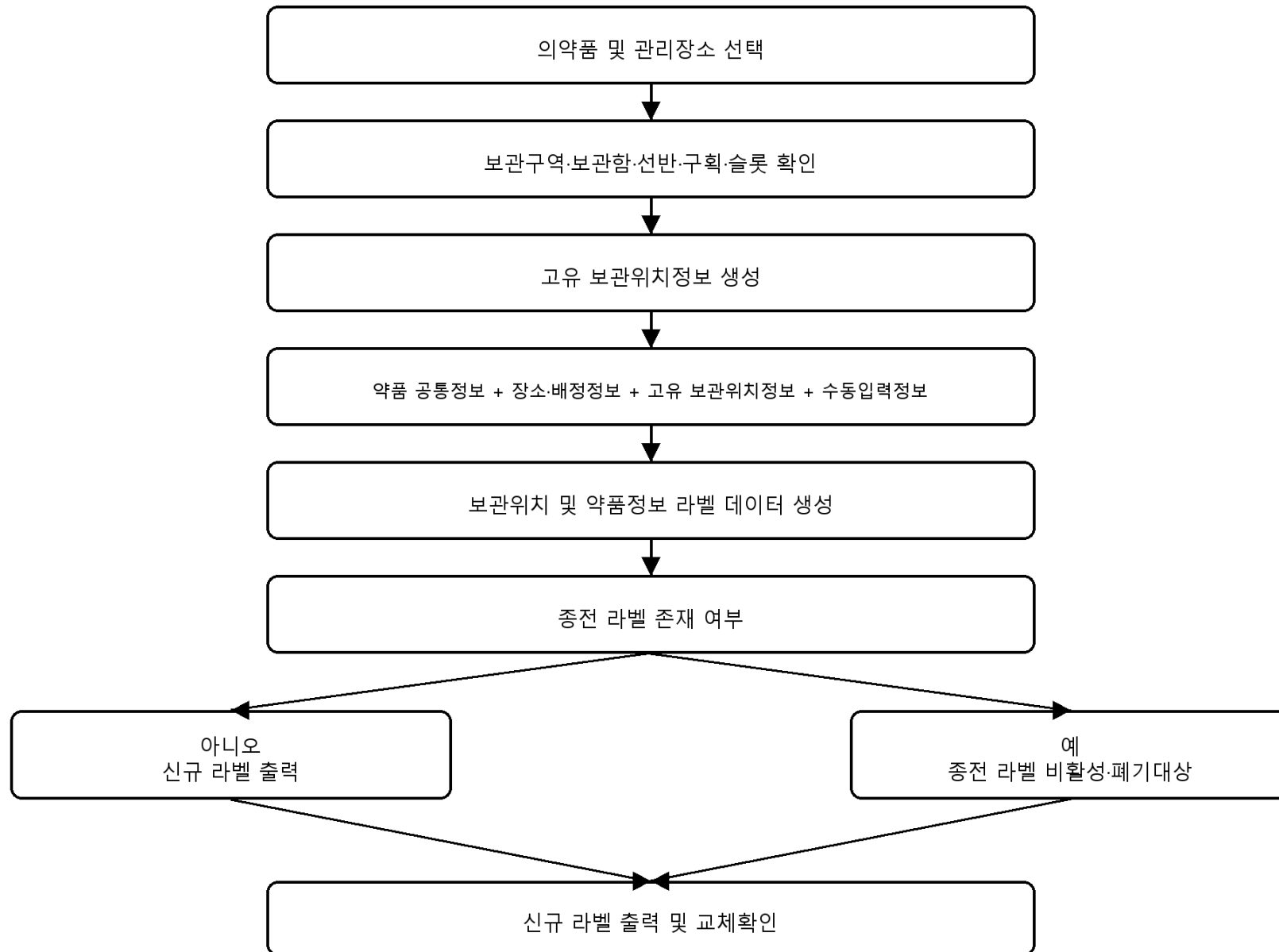
도 7. 고유 보관위치 및 라벨 관리 흐름도
