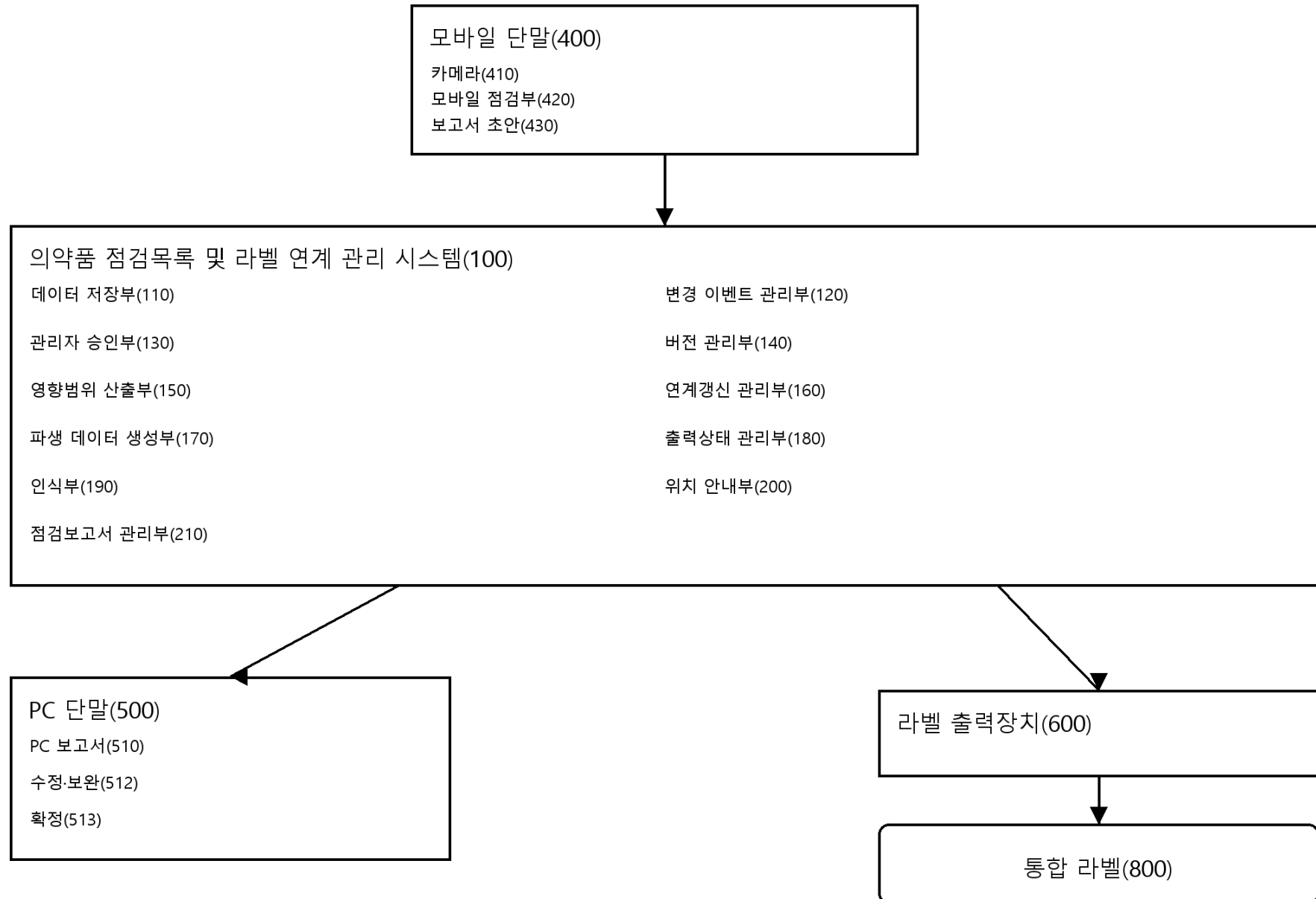
도 1. 전체 시스템 구성도
