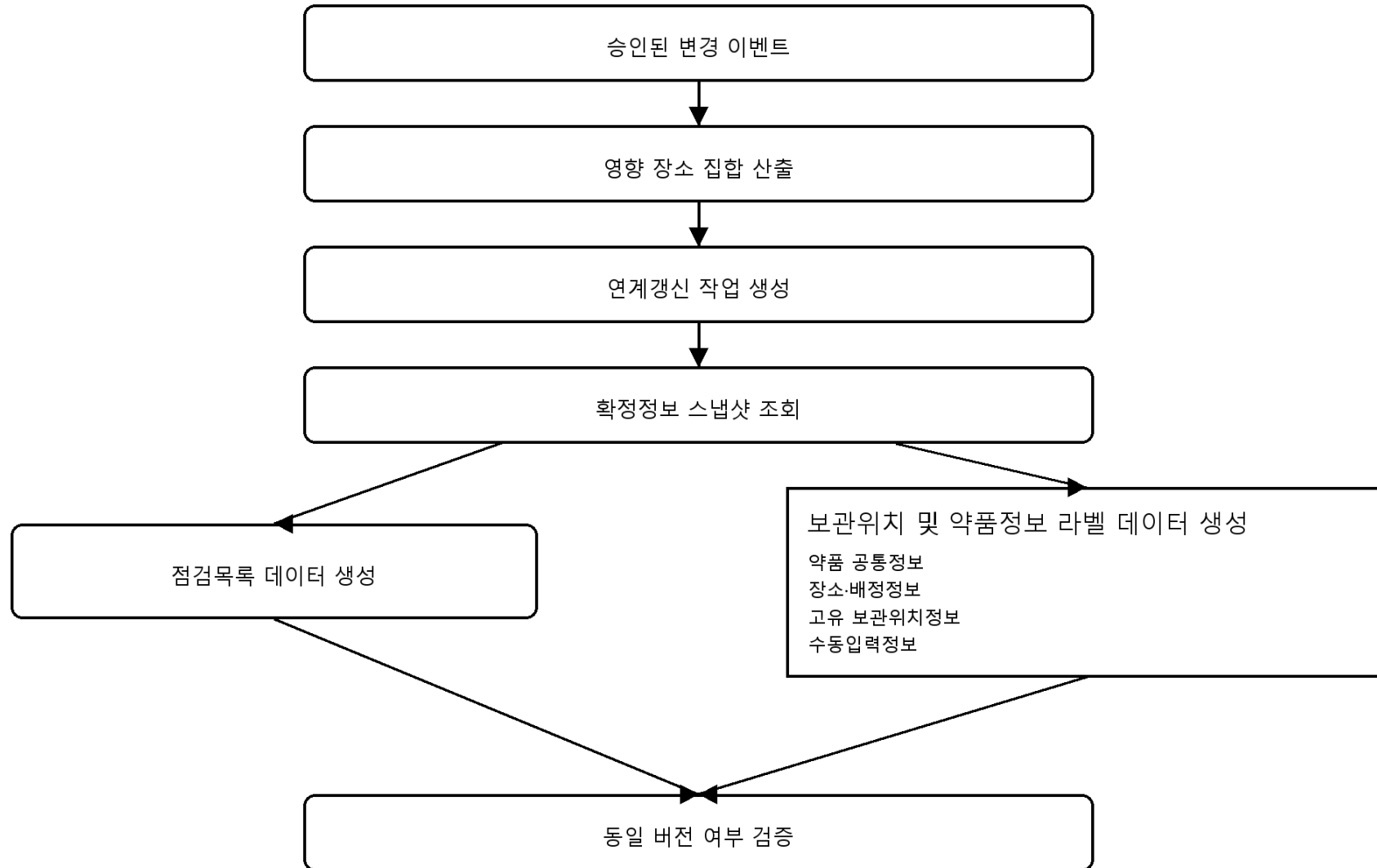
도 5. 연계갱신 흐름도
