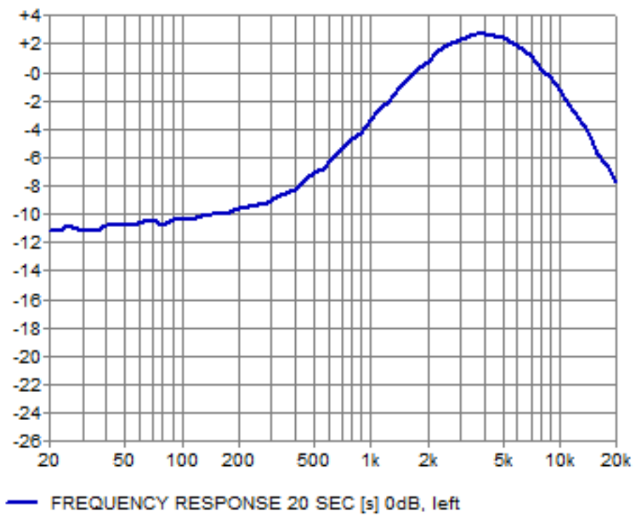
4KHz Low Q
