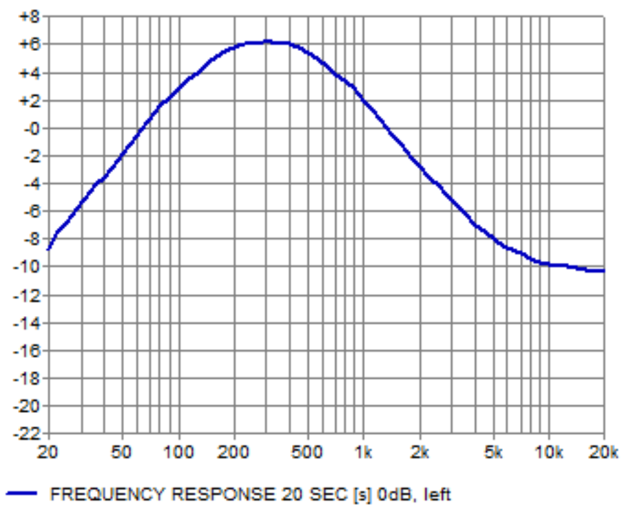
300Hz Boost
