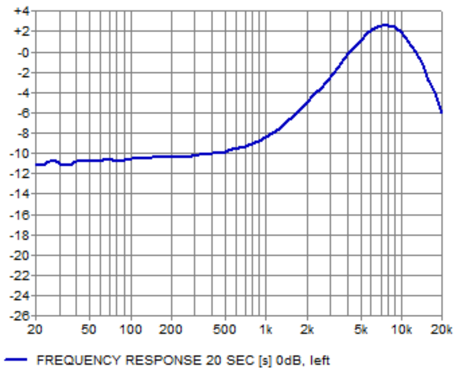
8KHz Low Q
