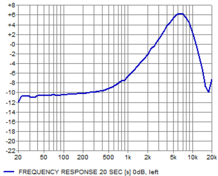
7KHz Boost
