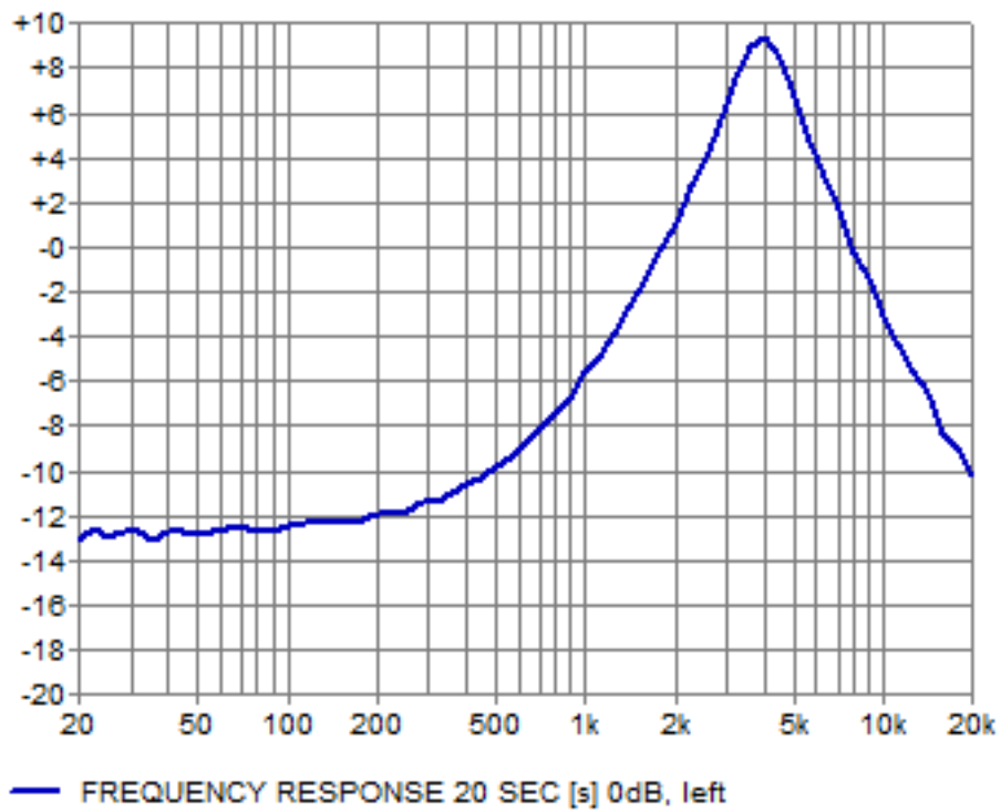
4KHz High Q
