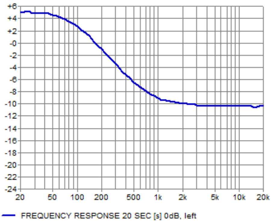
100Hz Boost
