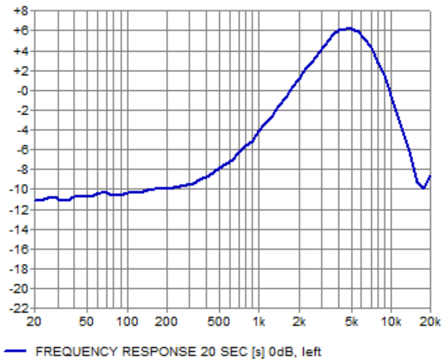
5KHz Boost
