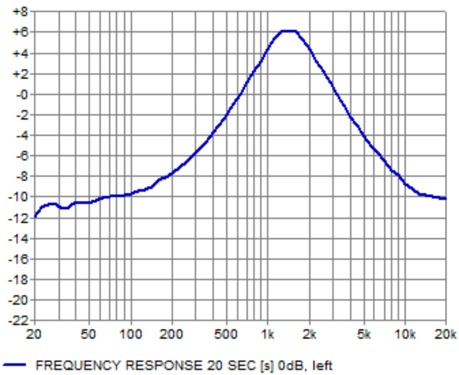
1K5KHz Boost
