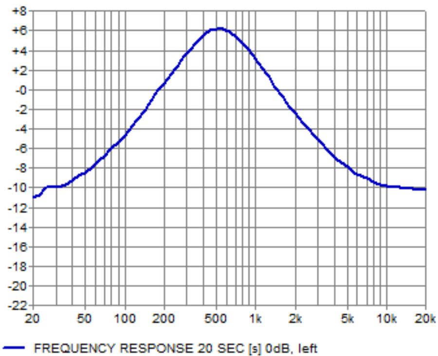
500Hz Boost
