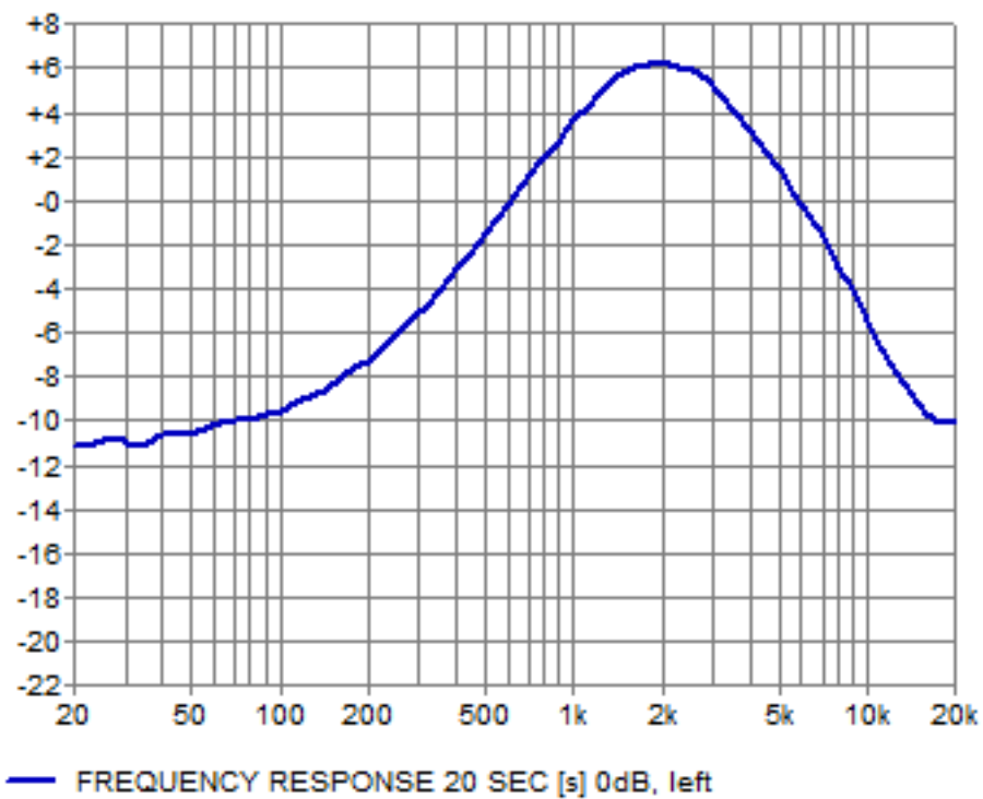
2KHz Boost
