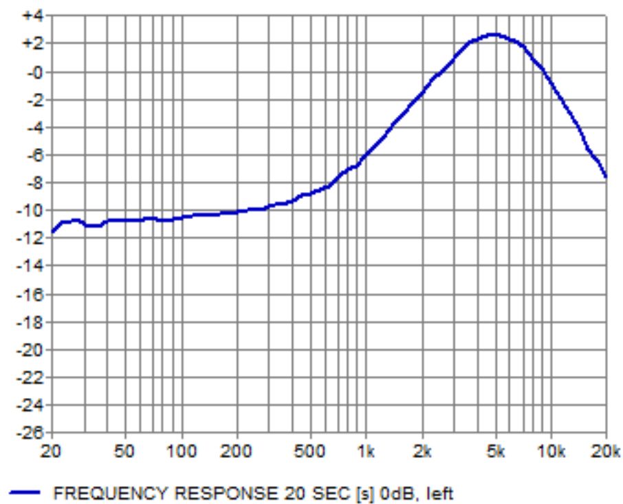
5KHz Low Q
