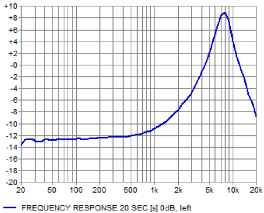
8KHz High Q
