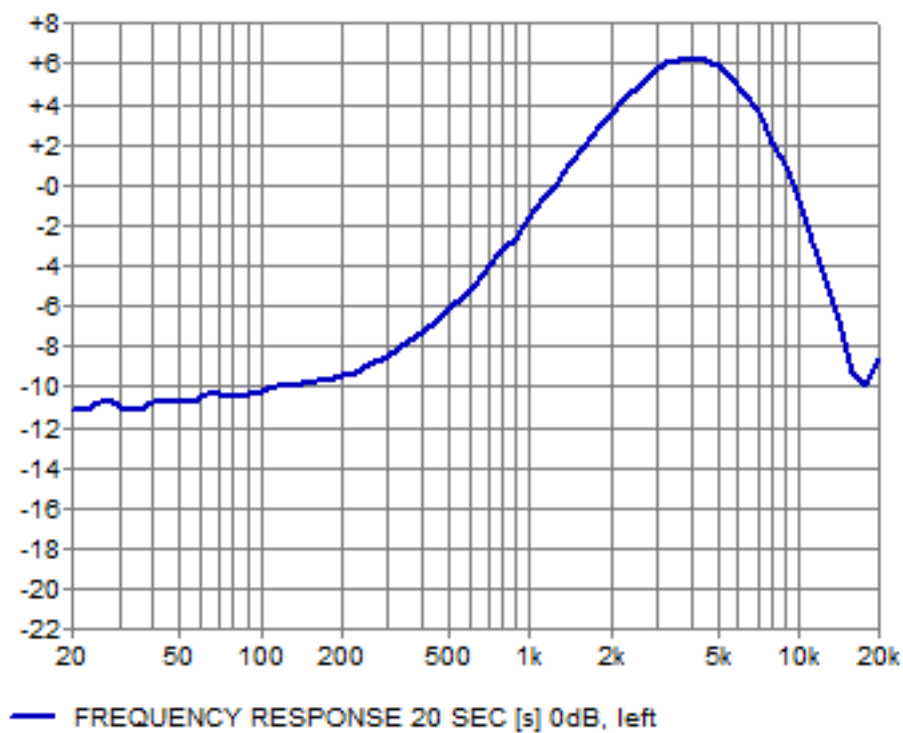
4KHz Boost
