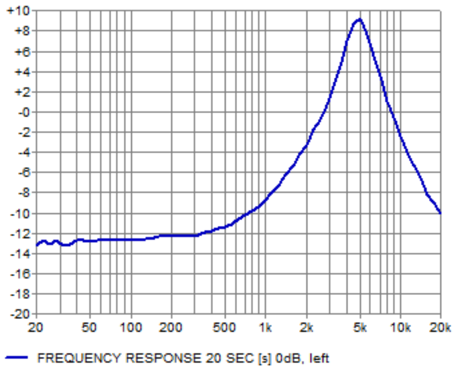
5KHz High Q
