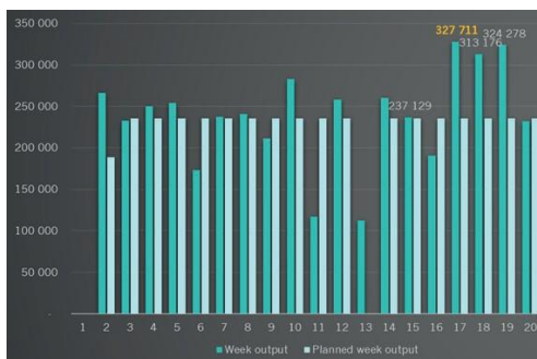
Продуктивність монтажної лінії CNP03 за тижнями
