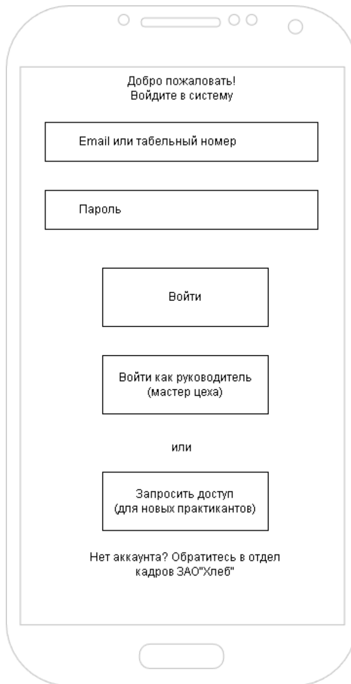
Рисунок 3 — Экран 1. Авторизация
