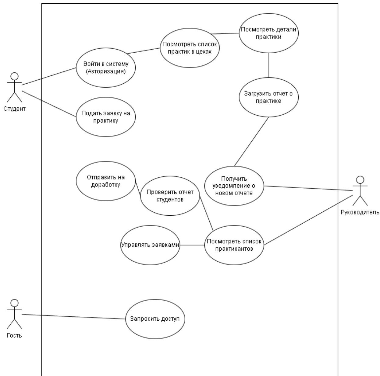
Рисунок 1 - Use Case диаграмма мобильного приложения для учета практики студентов на ЗАО «Хлеб»
