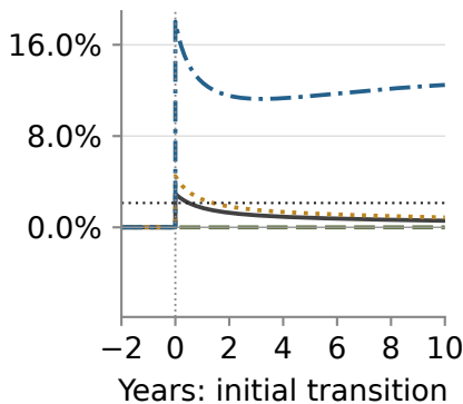
A. Output g_Y - (n + \gamma)
