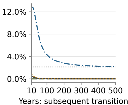
A. Output g_Y - (n + \gamma)
