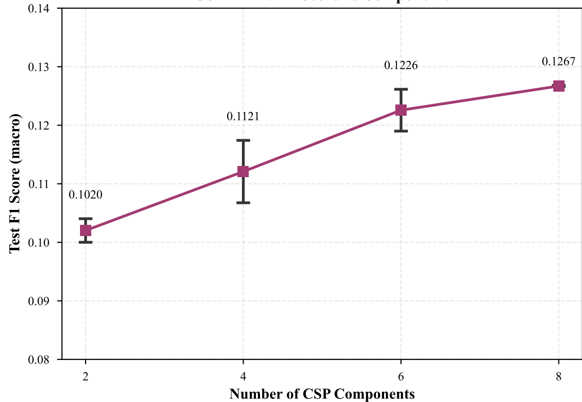
CSP+LDA: F1 Score vs Components
