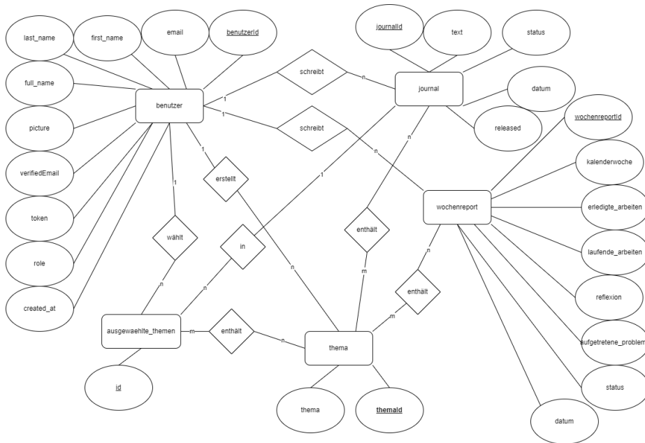
Abbildung 4: Das ERM-Diagramm
