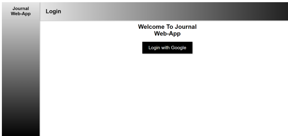
Abbildung 22: Login Seite
