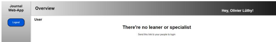
Abbildung 36: Overview-Seite
