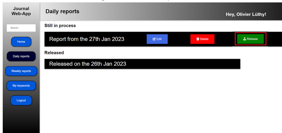
Abbildung 30: Tagesrapport veröffentlichen
