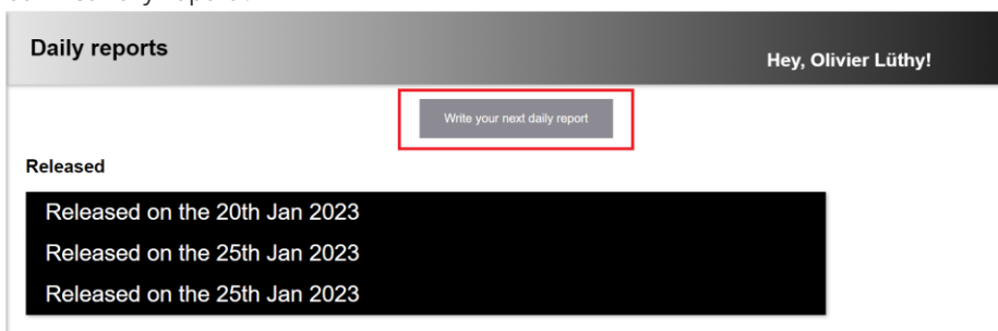
Abbildung 26: Tagesrapport hinzufügen
