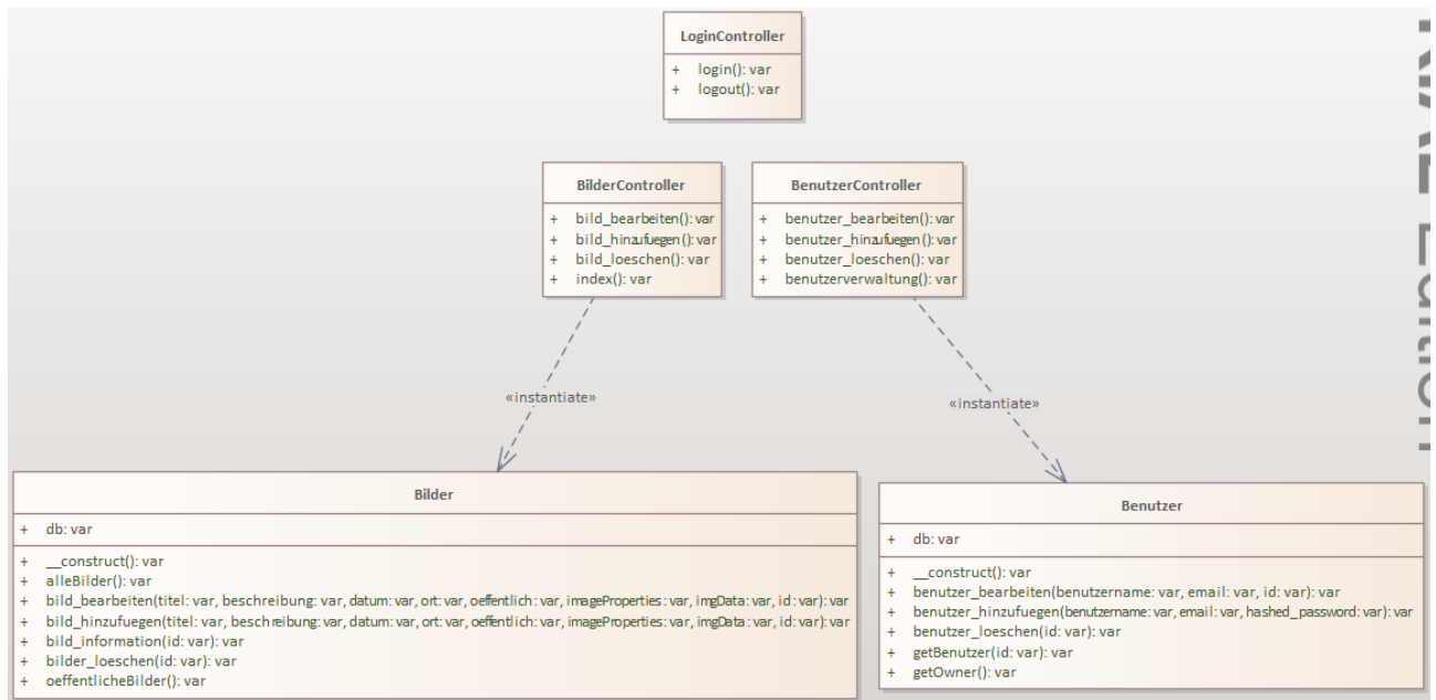
Abbildung 5: Klassendiagramm
