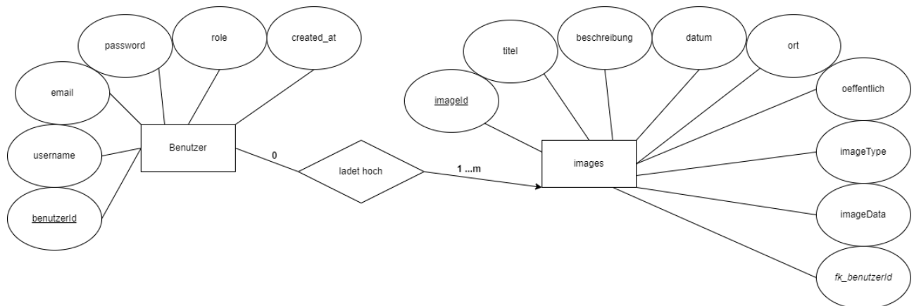
Abbildung 4: ERM-Diagramm
