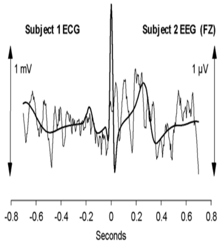
Figure 5. L'électricité du toucher. Formes d'onde moyennées montrant la détection de l'énergie électromagnétique générée par le cœur de la source dans l'EEG du sujet récepteur.
