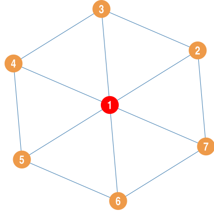
(d) Wheel Graph
