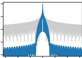
(d) Dolph-Chebyshev
