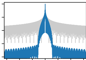
(d) Dolph-Chebyshev
