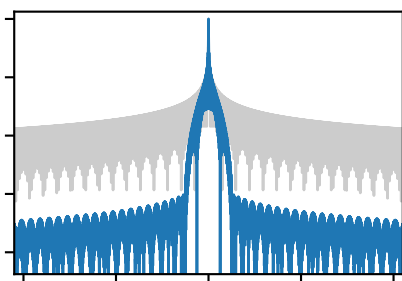
(d) Dolph–Chebyshev
