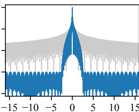
(d) Dolph-Chebyshev
