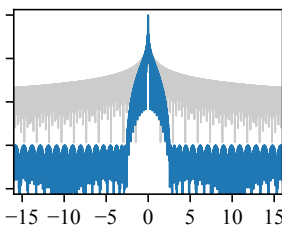
(d) Dolph-Chebyshev
