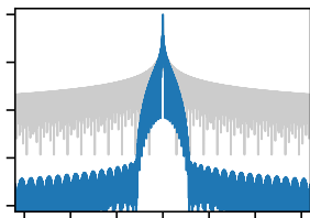
(d) Dolph-Chebyshev
