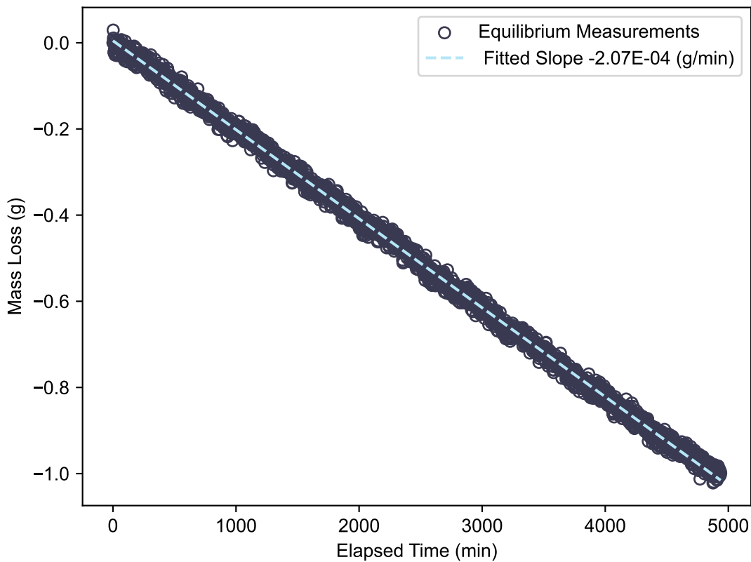
Cellulose_9
