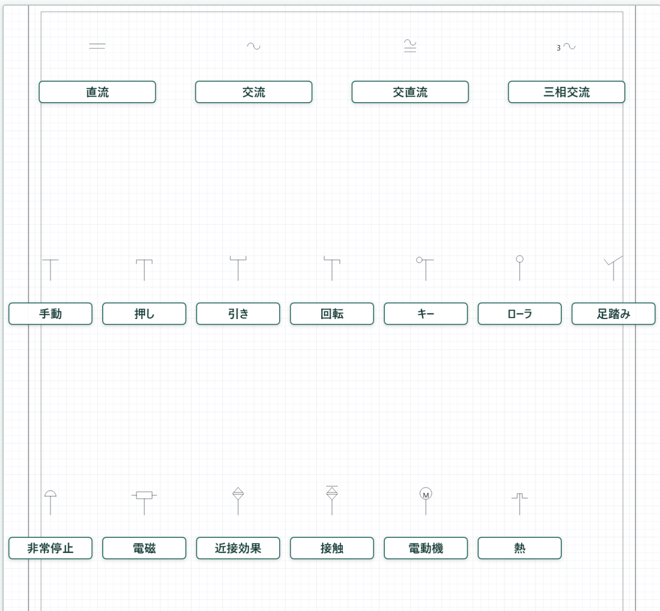
図21-20b 電流種別4種と操作機構13種の限定図記号。接点などの主記号へ組み合わせて使用します。
