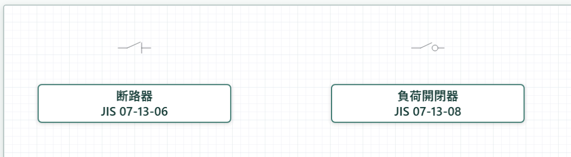
図21-19c 断路器 JIS 07-13-06と負荷開閉器 JIS 07-13-08。接点の円端子を描かず、固定接点側の止め棒または小円で区別します。
