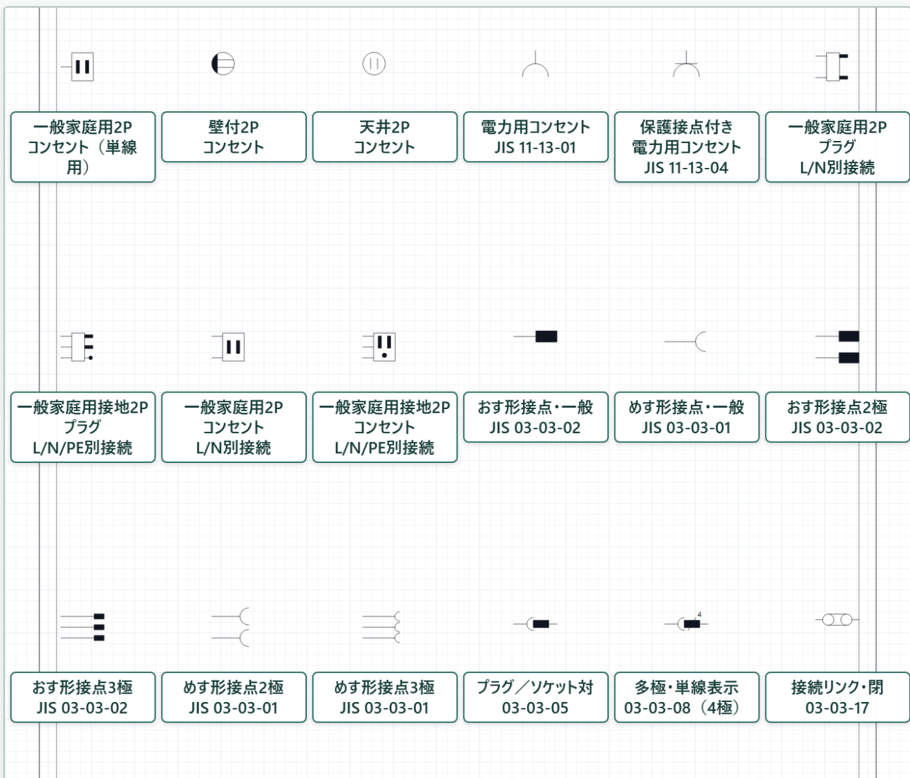
図21-15a コンセントのシンボルデザイン18種。一般家庭用2P外観、JIS C 0617の1極・2極・3極接点、プラグ及びソケット対、多極単線表示、接続リンクを比較できます。
