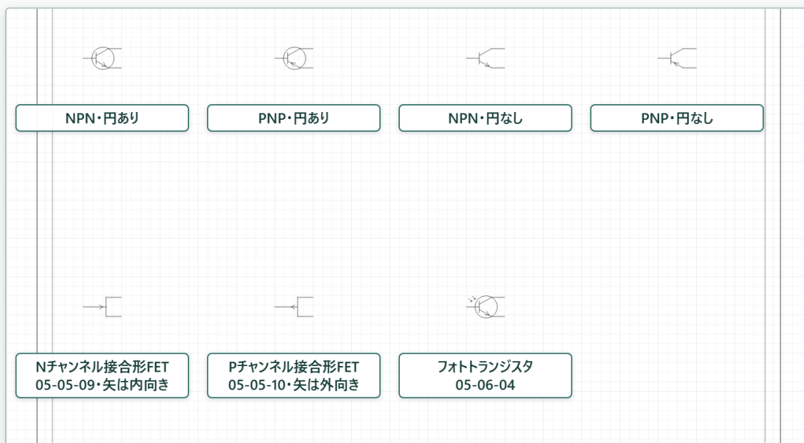
図21-19a トランジスタ7種。N/Pチャンネル接合形FETを含み、N形はゲート矢印が内向き、P形は外向きです。
