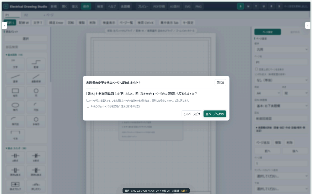
図5-2 表題欄を変更したときの確認。現在ページだけに残すか、全ページへ反映するかを選び、セッション中の選択を記憶できます。
