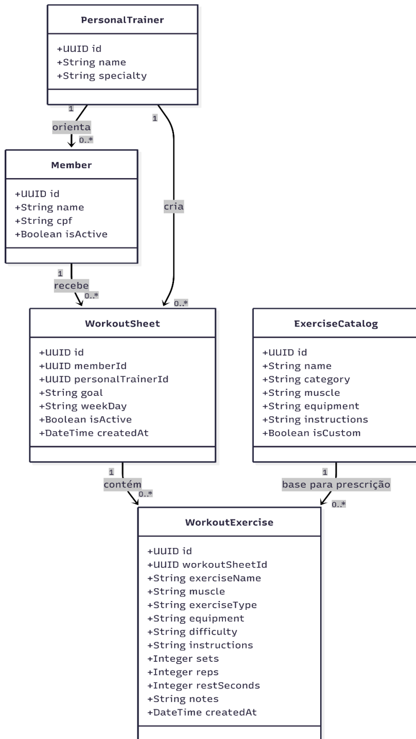
Diagrama de ER do Contexto
