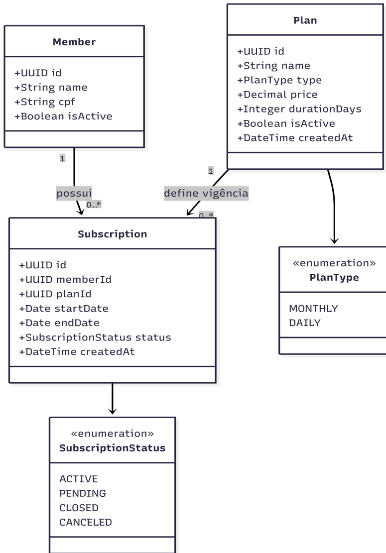
Diagrama de ER do Contexto
