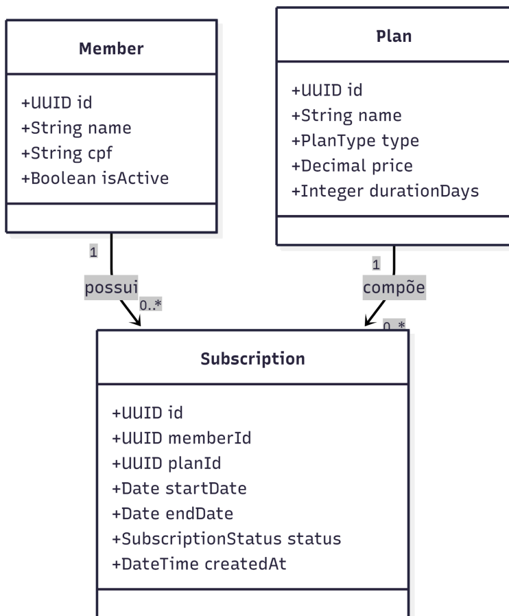
Diagrama de ER do Contexto
