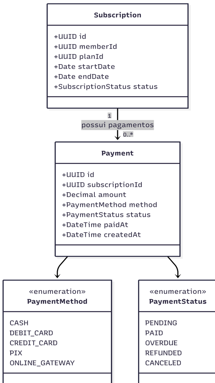
Diagrama de ER do Contexto
