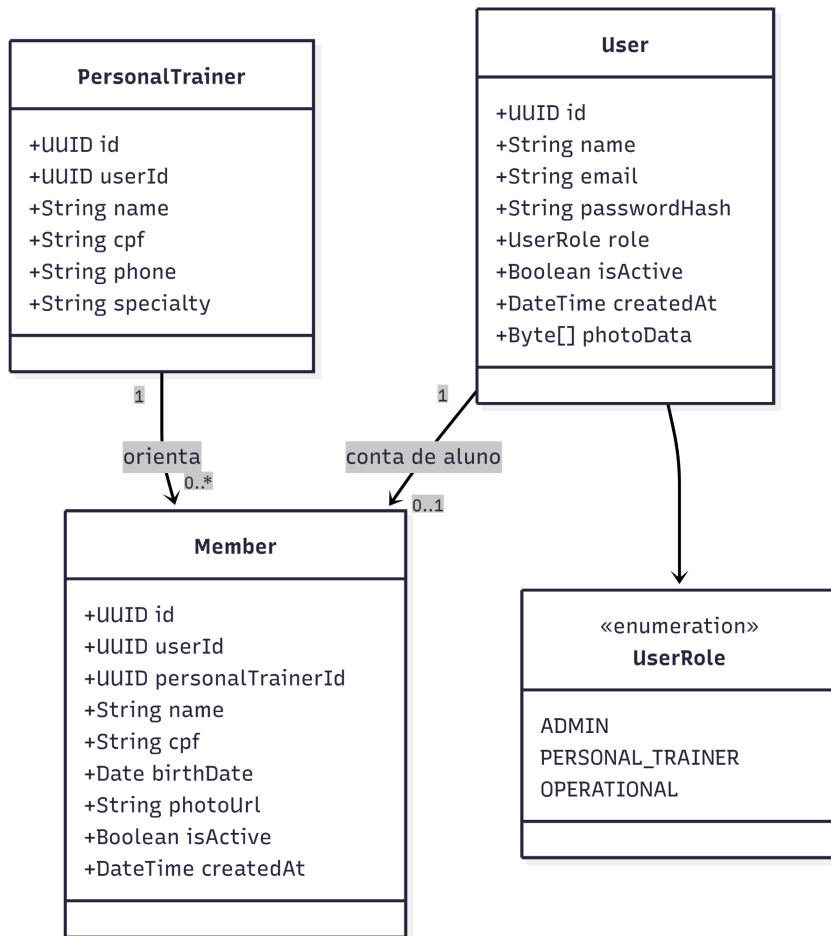
Diagrama de ER do Contexto
