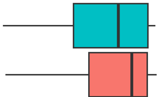
Borzoï Prime
