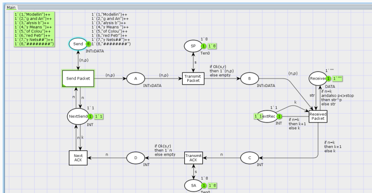
Рис. 6: Модель простого протокола передачи данных
