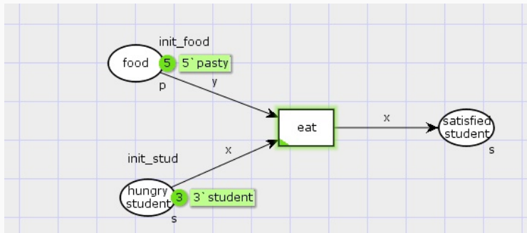
Рис. 2: Граф сети модели «Накорми студентов»
