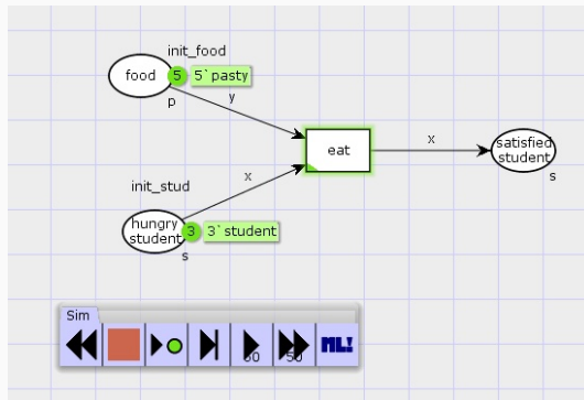
Рис. 4: До запуска симуляции
