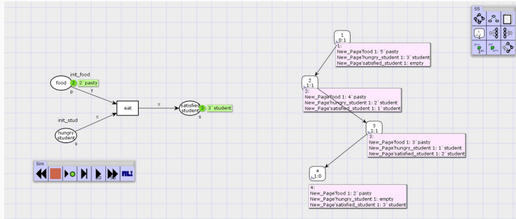
Рис. 6: Пространство состояний для модели «Накорми студентов»
