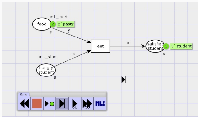
Рис. 5: После запуска симуляции
