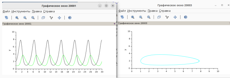
Рис. 11: Динамика изменения численности хищников и жертв, и фазовый портрет
