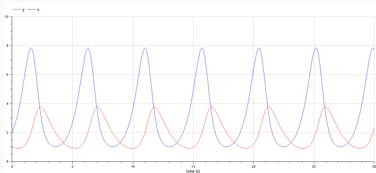
Рис. 14: Динамика изменения численности хищников и жертв модели при a = 2 , b = 1 , c = 0.3 , d = 1 , x(0) = 2 , y(0) = 1 в OpenModelica
