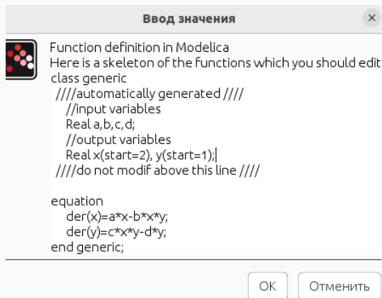
Рис. 9: Листинг для блока Modelica
