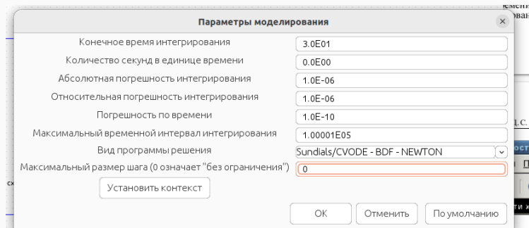
Рис. 5: Задание конечного времени интегрирования
