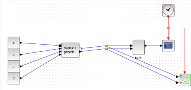
Рис. 10: Модель «хищник-жертва» с помощью блока Modelica
