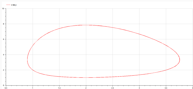
Рис. 13: Фазовый портрет модели при a = 2 , b = 1 , c = 0.3 , d = 1 , x(0) = 2 , y(0) = 1 в OpenModelica
