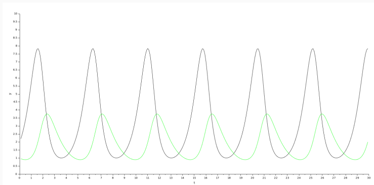
Рис. 6: Динамика изменения численности хищников и жертв модели при a = 2 , b = 1 , c = 0.3 , d = 1 , x(0) = 2 , y(0) = 1
