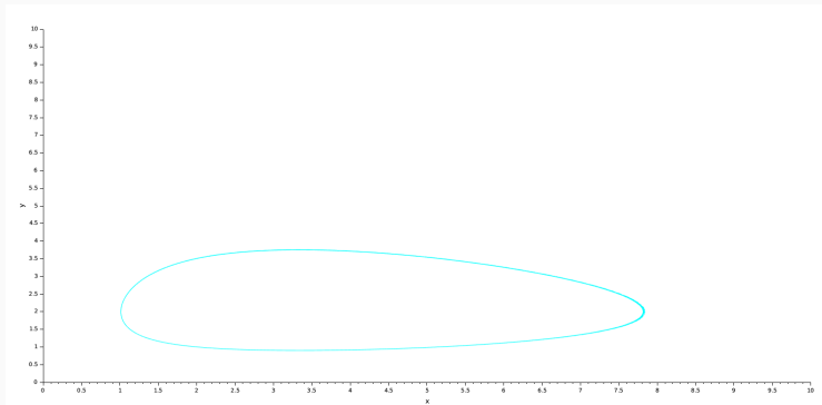
Рис. 7: Фазовый портрет модели при a = 2, b = 1, c = 0.3, d = 1, x(0) = 2, y(0) = 1
