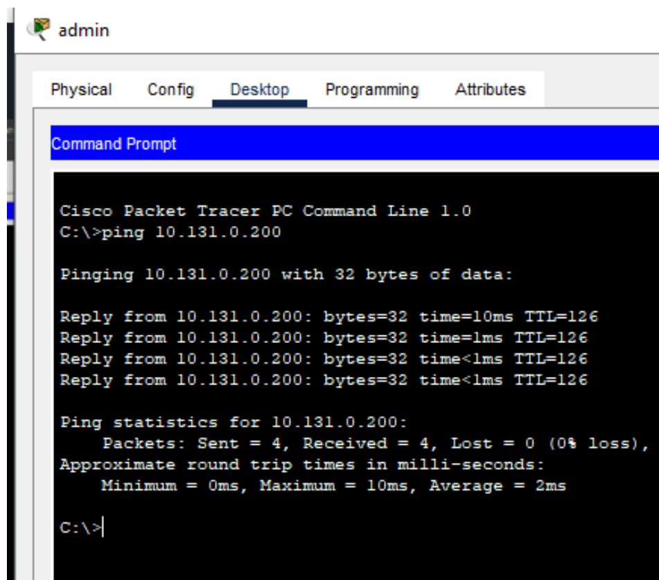
Рис. 5.23: Пингование сети
