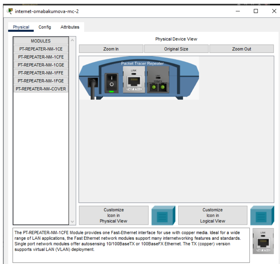
Рис. 5.2: Замена модулей на internet-omabakumova-mc-2
