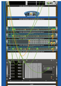
Рис. 13: Перемещение msk-pavlovskaya-mc-1, остался только msk-donskaya-mc-1
