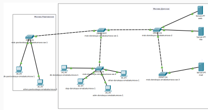
Рис. 1: Размещение коммутаторов и конечных устройств согласно схеме сети L1
