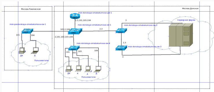
Рис. 3: Схема VLAN сети (Layer 2)
