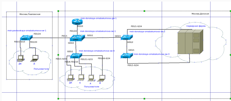
Рис. 1: Физические устройства сети с номерами портов (Layer 1)
