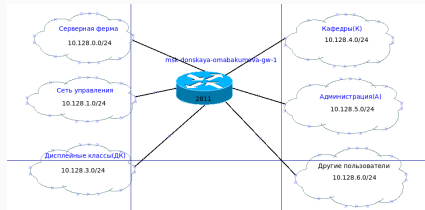
Рис. 4: Схема маршрутизации сети (Layer 3)
