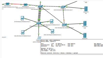
Рис. 5: Размещение ноутбука администратора в сети
