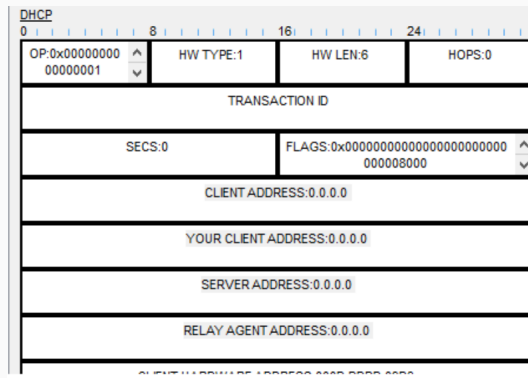
Рис. 26: Информация о PDU
