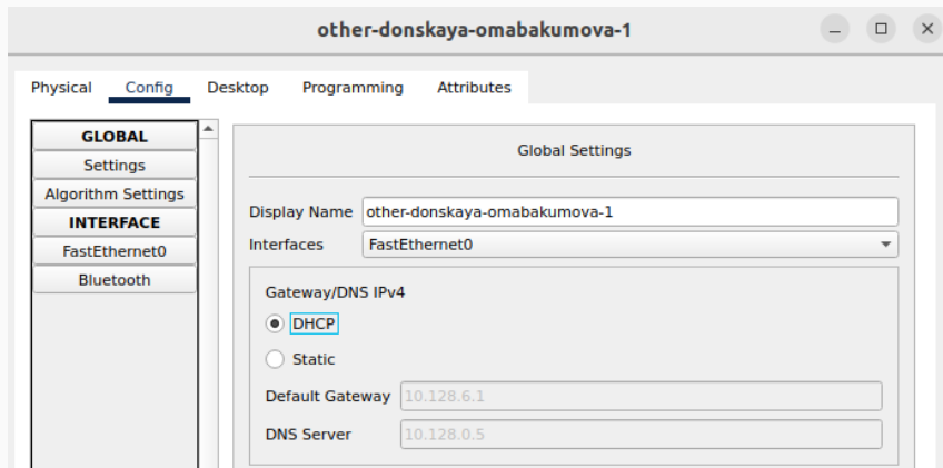
Рис. 17: Настройка динамического распределения на other-donskaya-omabakumova-1
