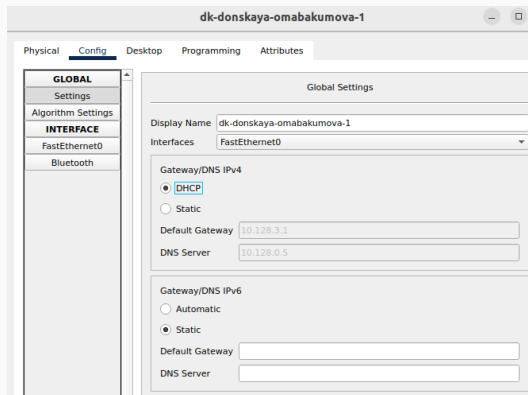
Рис. 12: Смена распределения на динамическое
