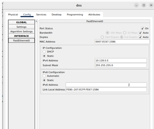
Рис. 3: Указание адреса самого сервера и его маски
