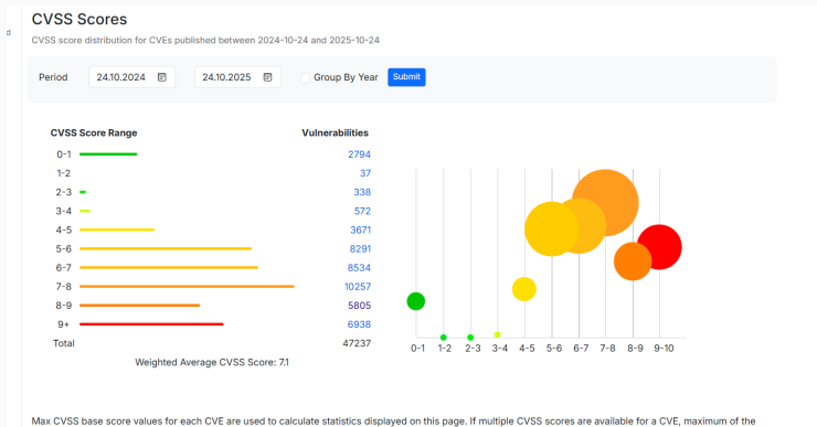
Рис. 8: Страница CVSS Scores
