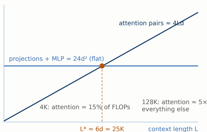
Per-token FLOPs per layer (7B geometry)
