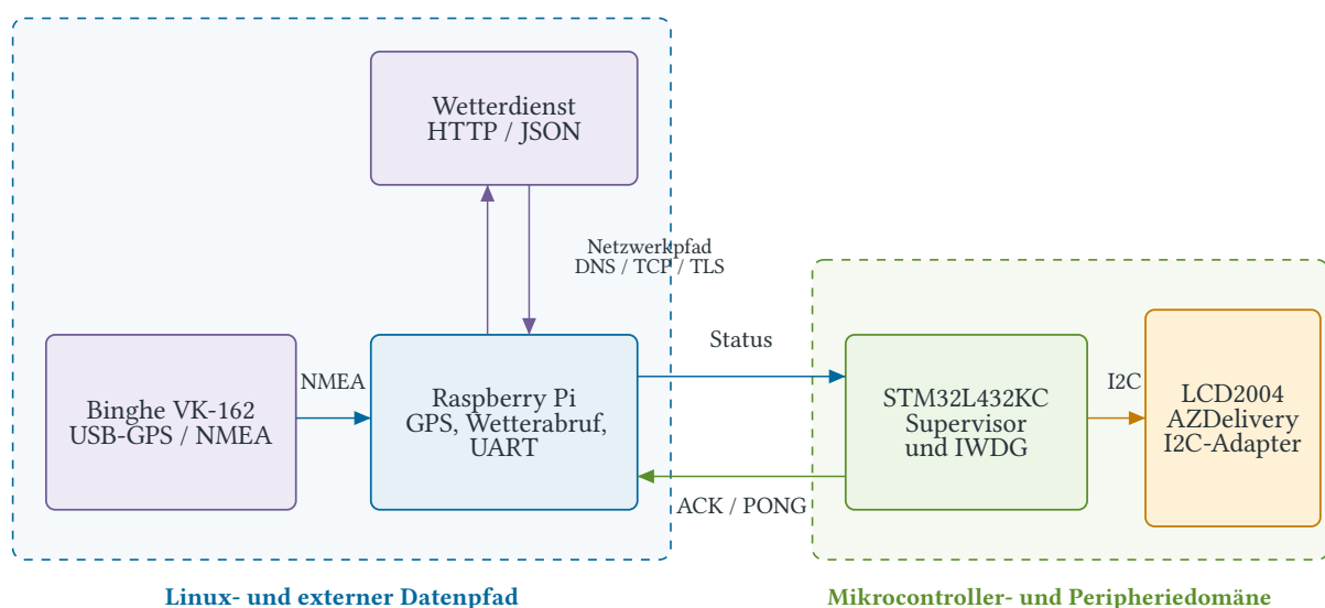
Abbildung 3.1: Gesamtarchitektur und wesentliche Datenpfade des Versuchssystems
