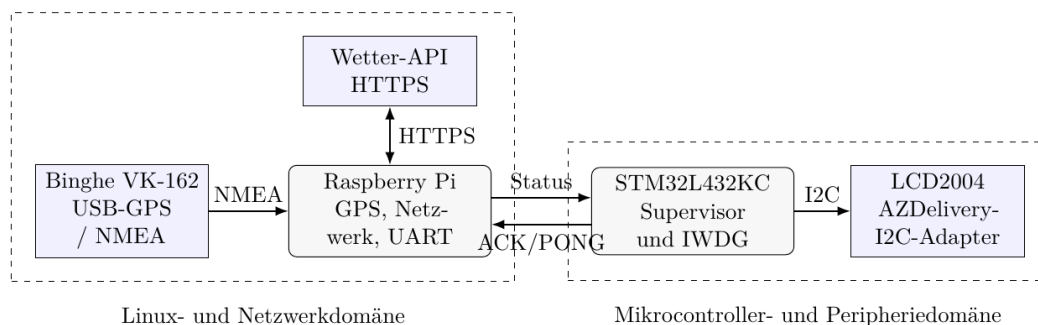
Abbildung 3.1: Gesamtarchitektur und wesentliche Datenpfade des Versuchssystems
