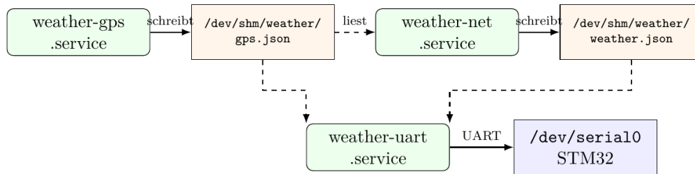
Abbildung 3.2: Entkopplung der Raspberry-Pi-Dienste über atomar aktualisierte Zustandsdateien
