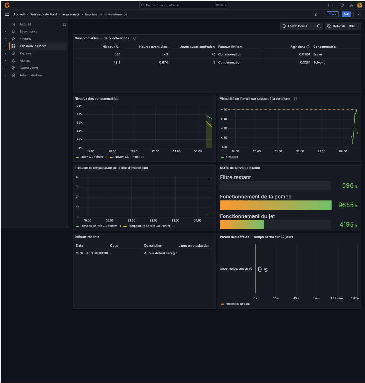
FIGURE 7.2 – Tableau de bord de maintenance : consommables, tendances et défauts
