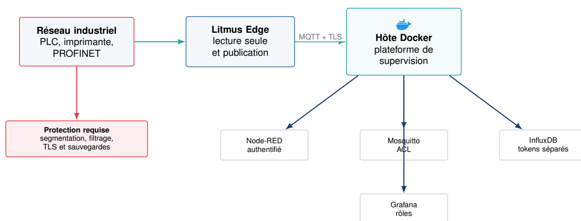
FIGURE 10.1 – Déploiement proposé et mesures à appliquer avant le raccordement
