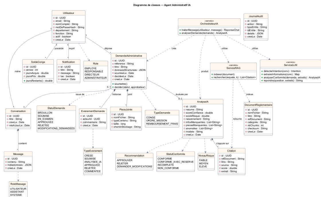
Figure 2.2. Diagramme de classes du domaine
