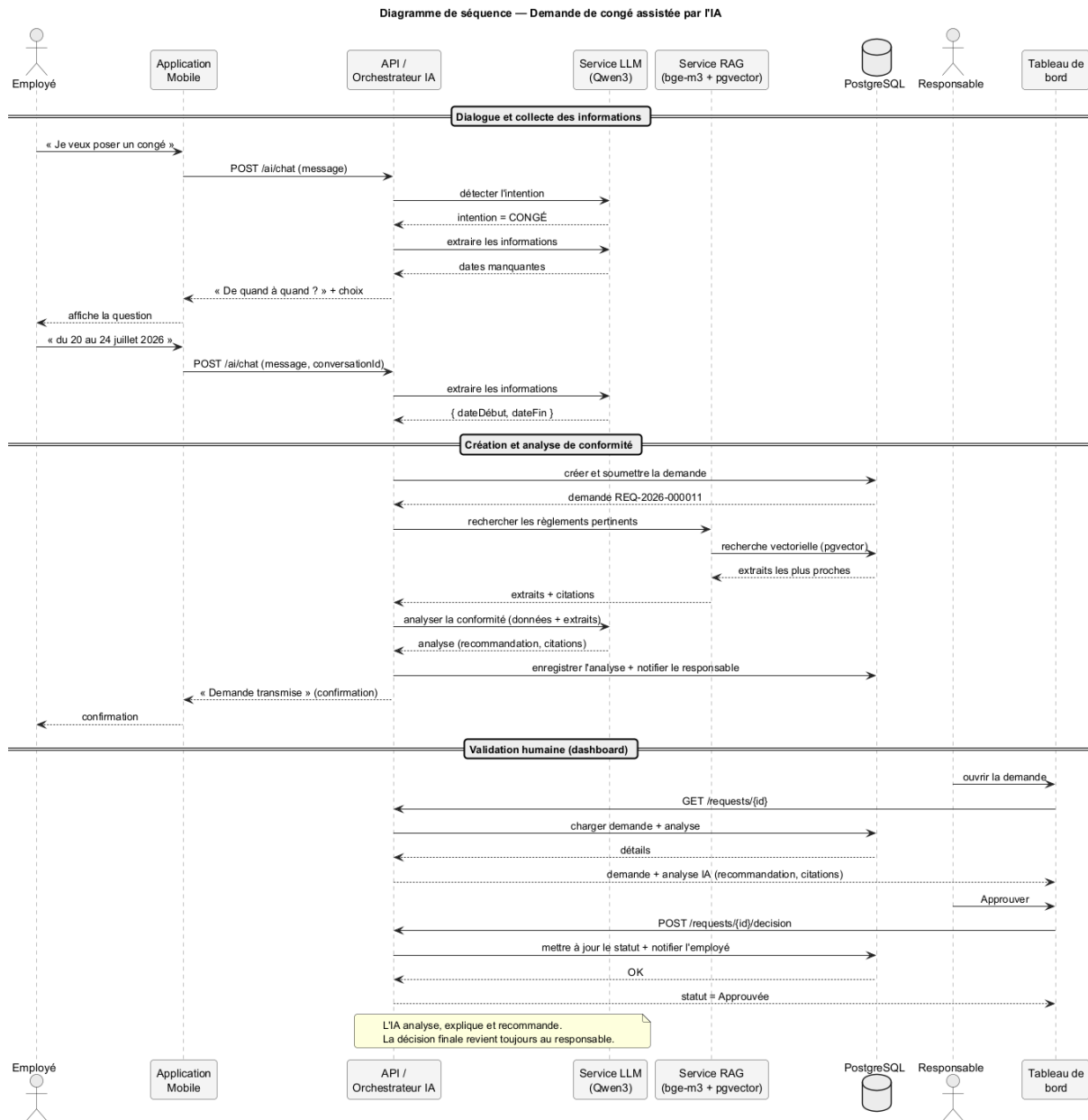
Figure 2.3. Diagramme de séquence : demande assistée puis validation
