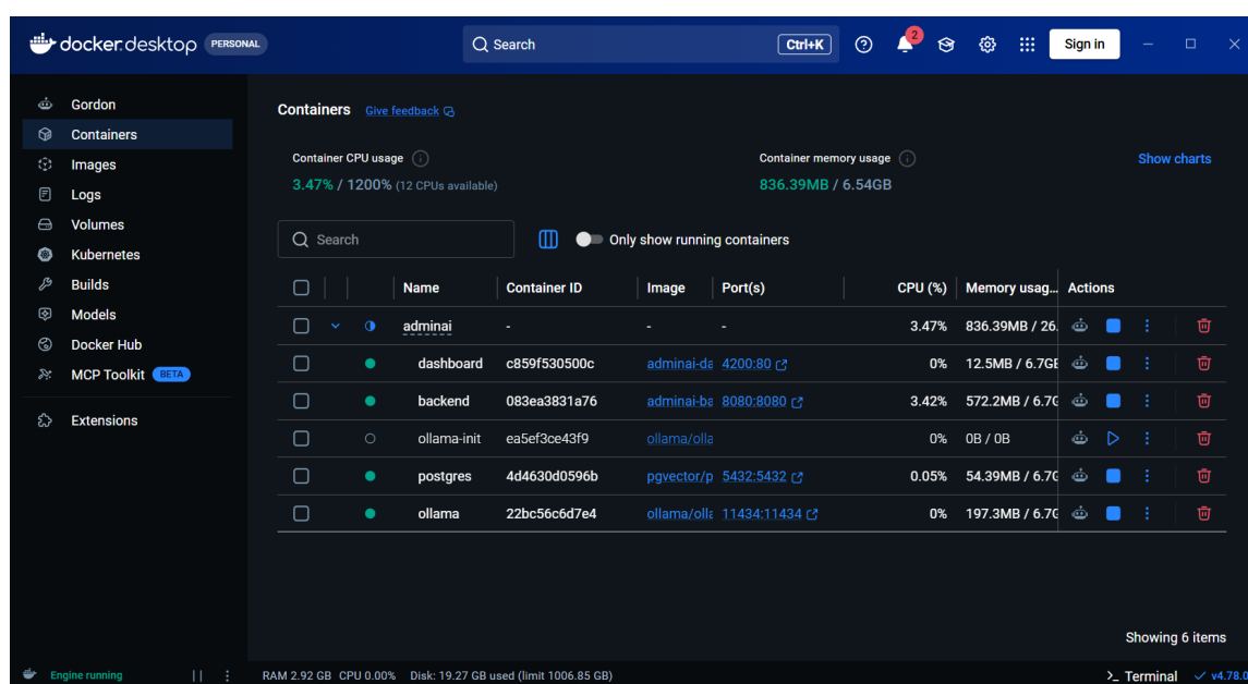
Figure 3.2. Pile applicative conteneurisée en cours d'exécution
