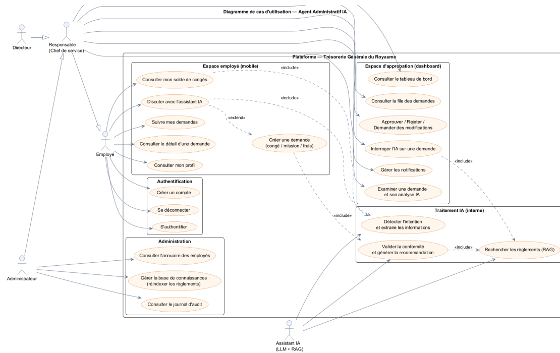
Figure 2.1. Diagramme de cas d'utilisation
