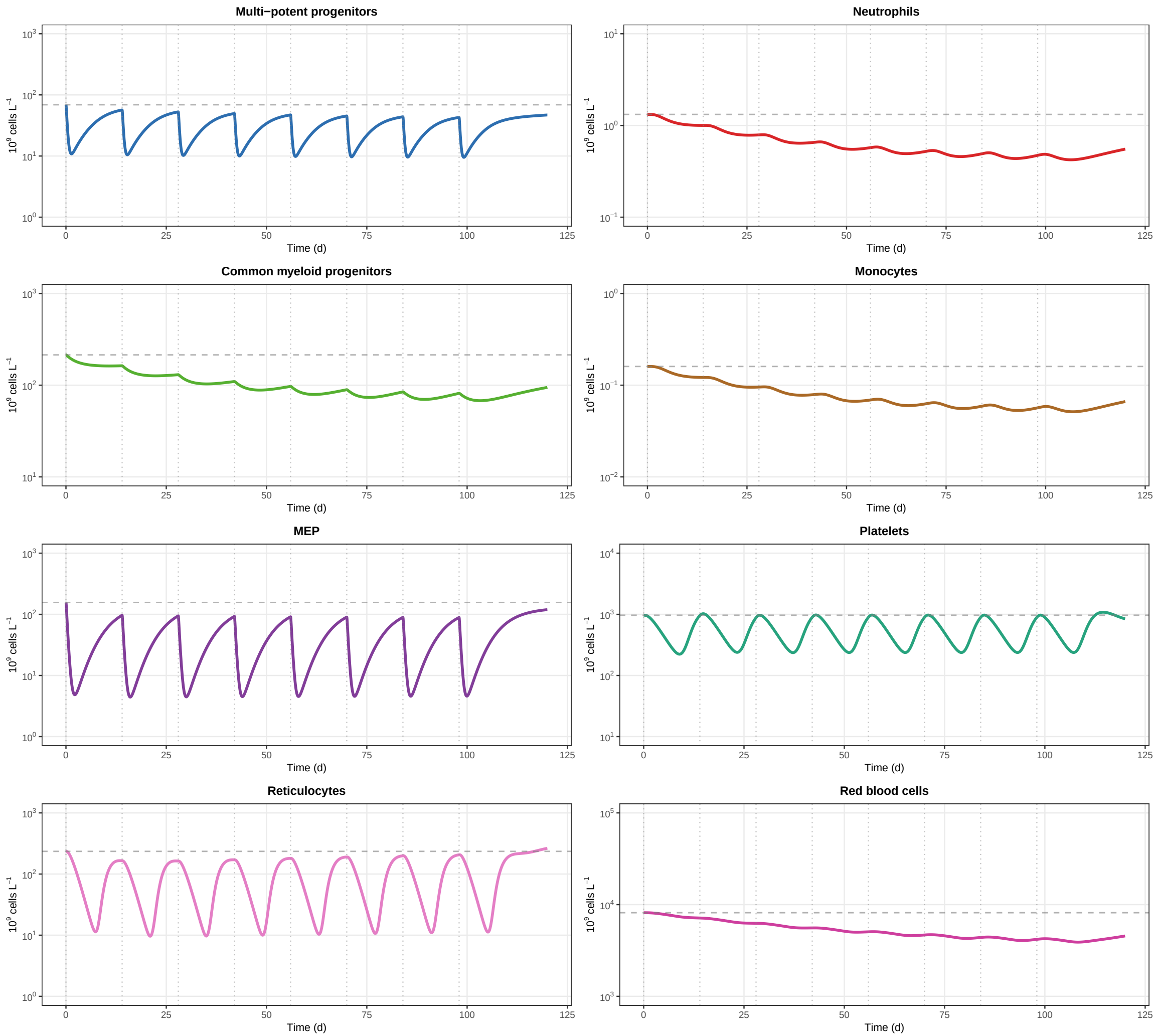
Figure 3 – Carboplatin 40 mg/kg Q14D x 8 (simulation)
