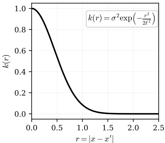
RBF kernel
