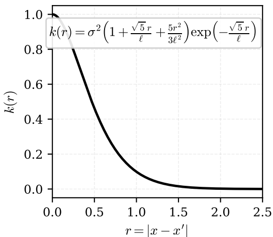
Matérn 5/2 kernel
