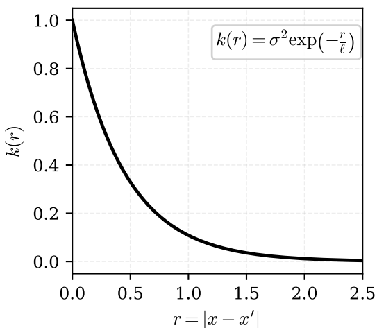
Matérn 1/2 kernel
