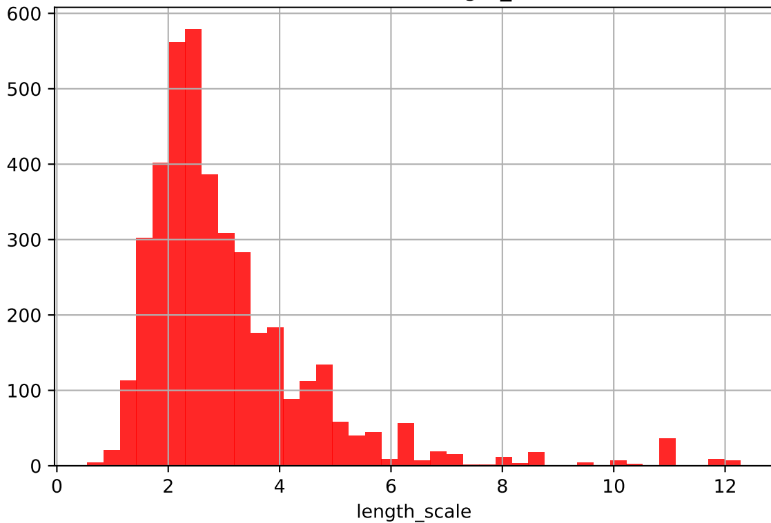
Posterior of GP length_scale
