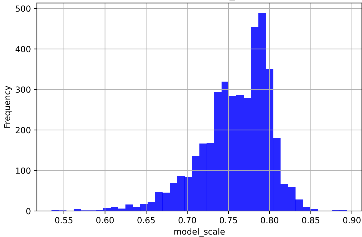
Posterior of model_scale
