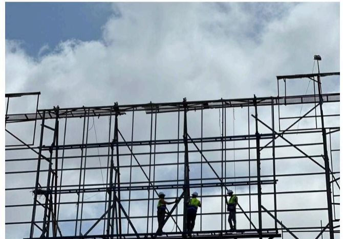
التنفيذ تركيب الهيكل المعدني للشاشة
