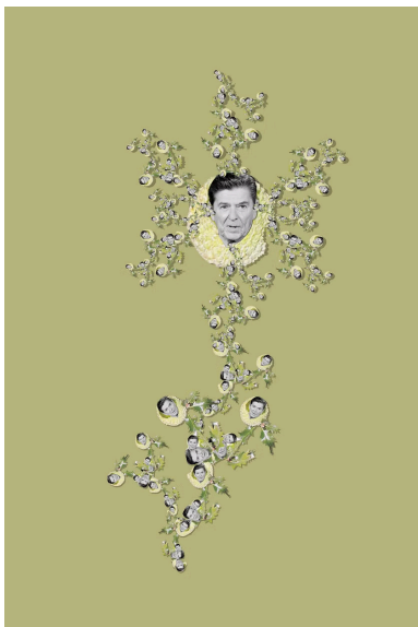
رقم (٠٣) IMG (03)
