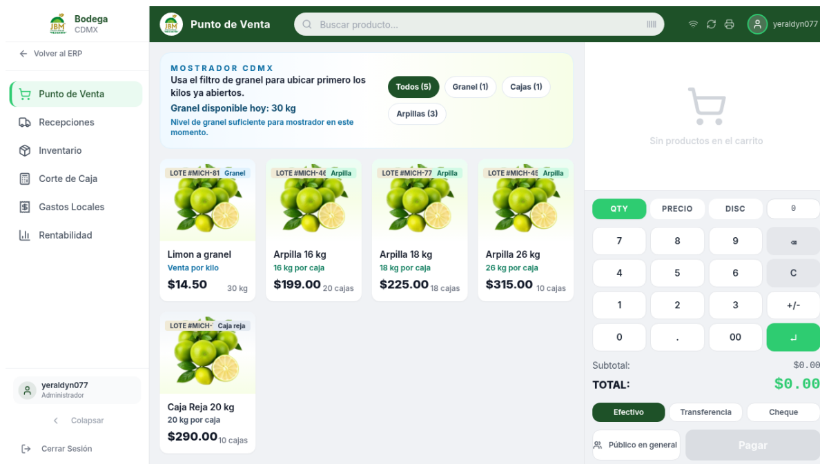
Punto de Venta CDMX — catálogo de productos, carrito y numpad
