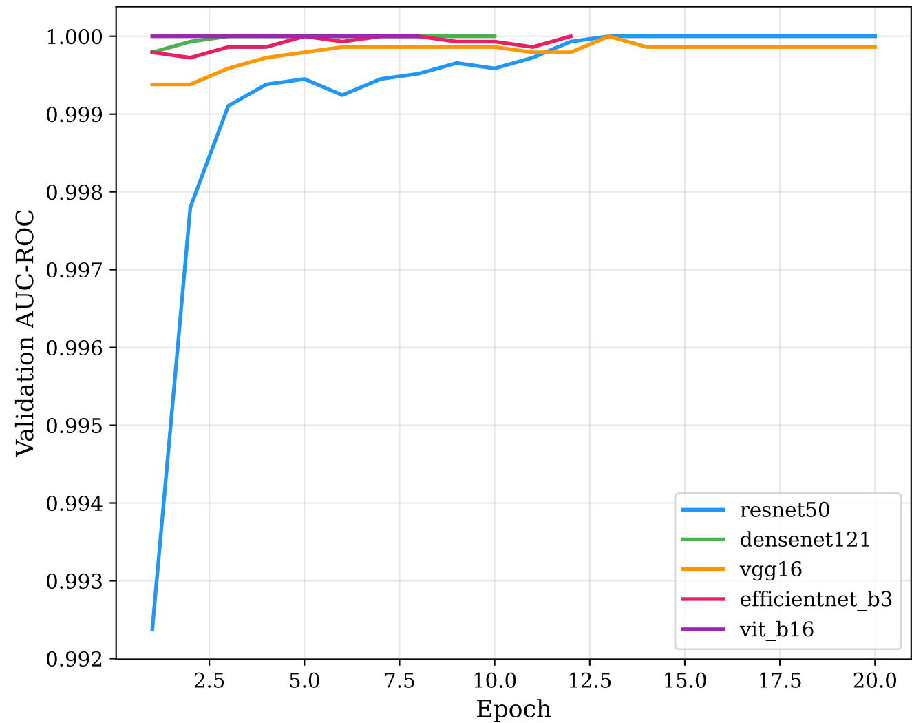
Validation AUC Curves
