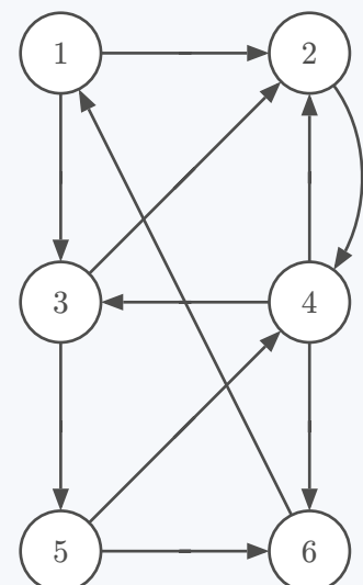
Markov-Kette
