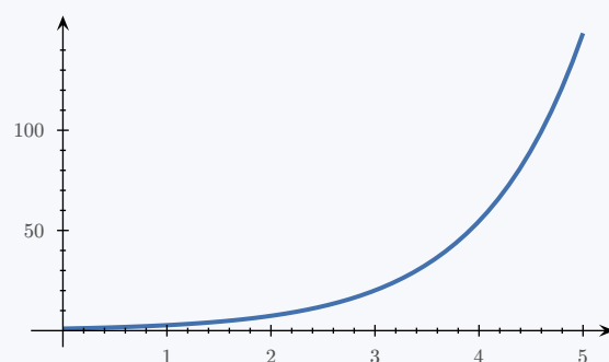
Beispiel 8 : f(x) = e^x
