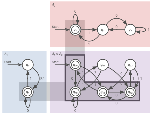
Symmetrische Differenz L(A_1) \Delta L(A_2)
