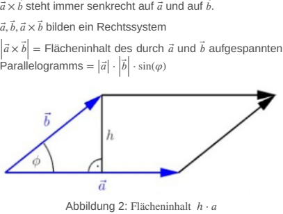
Abbildung 2: Flächeninhalt h \cdot a
