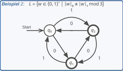
Beispiel 2: L = \{w \in \{0, 1\}^* \mid |w|_0 \not\equiv |w|_1 \pmod 3\}
