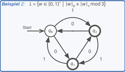
Beispiel 2: L = \{w \in \{0, 1\}^* \mid |w|_0 \equiv |w|_1 \pmod 3\}
