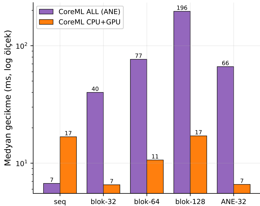
(b) CoreML gecikmesi
