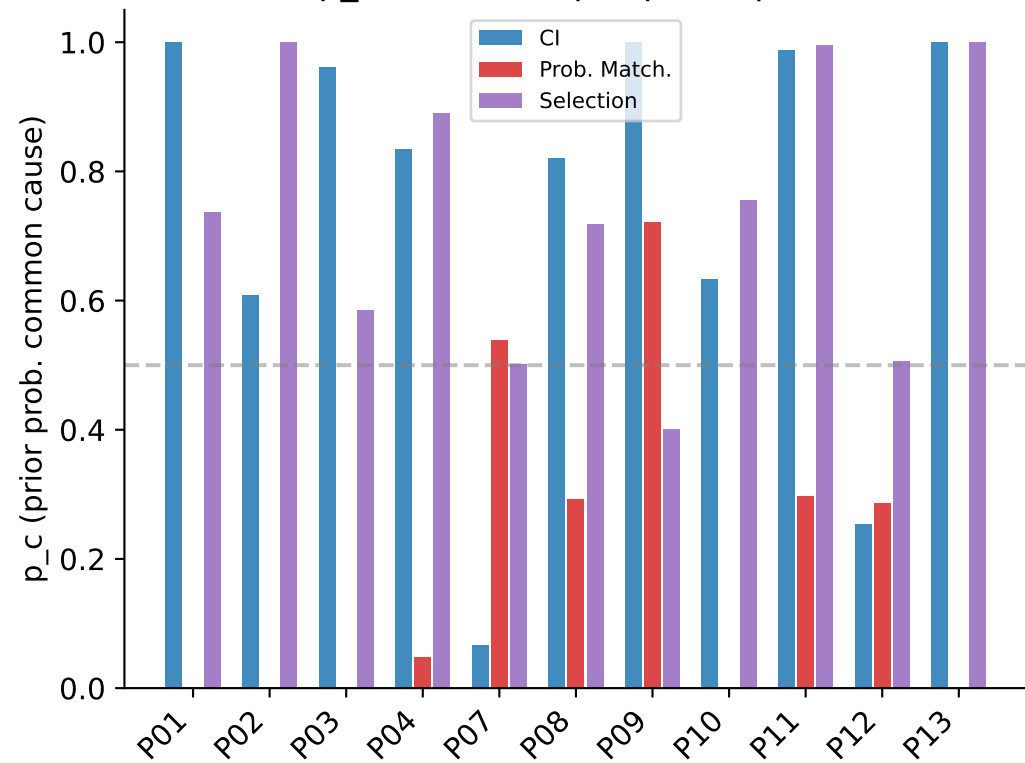
p_c estimates per participant
