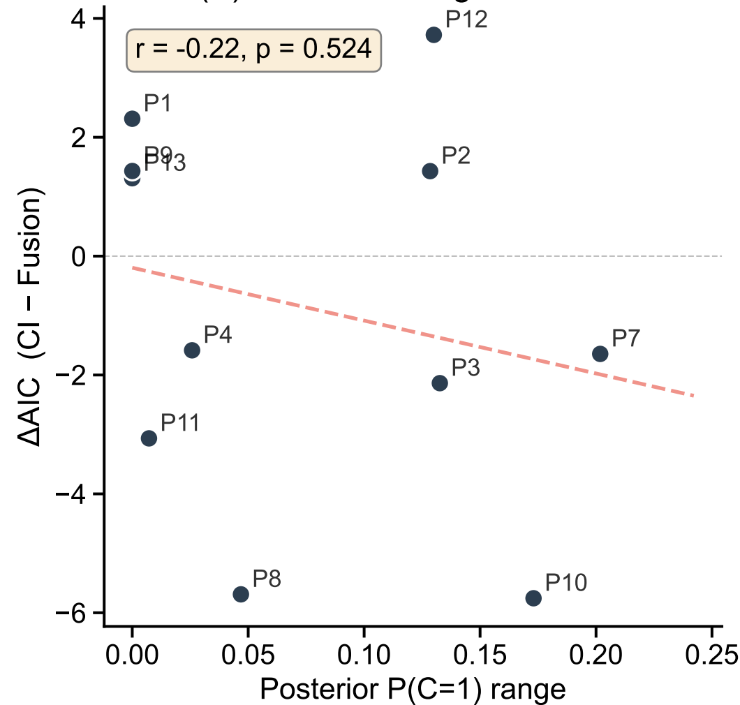
(B) Posterior range vs. \Delta AIC
