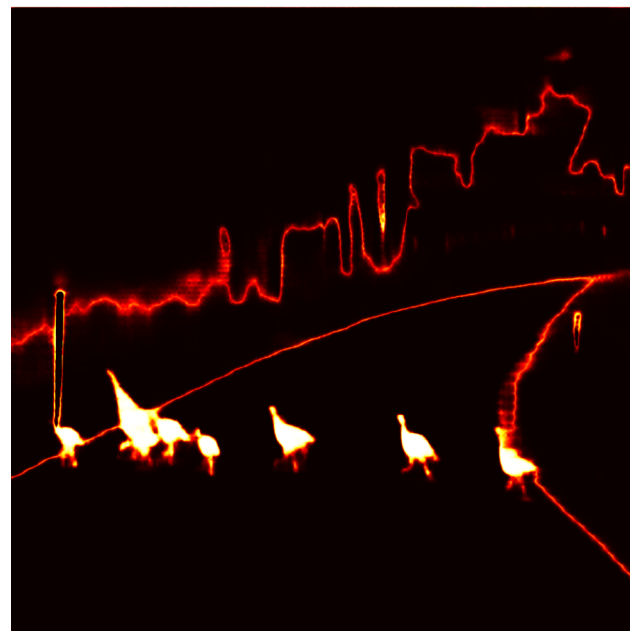
MaxLogit
