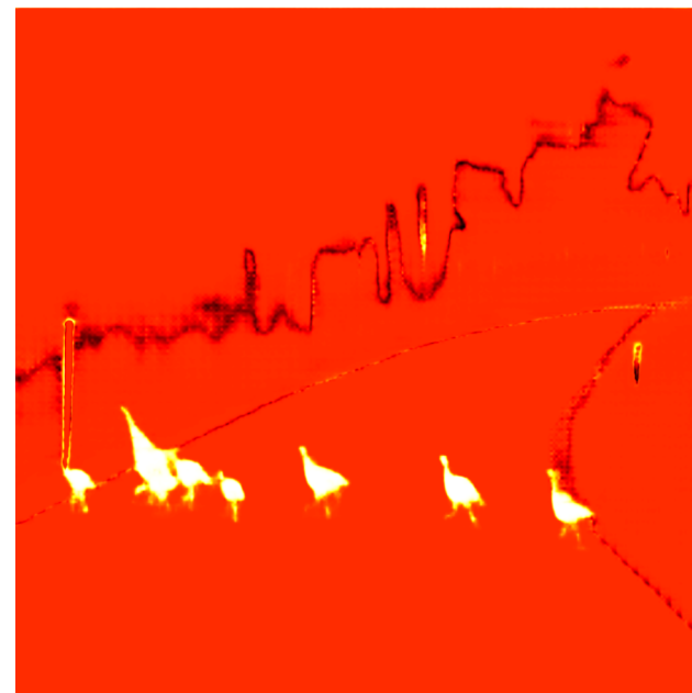
RbA
