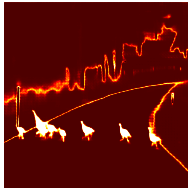
MaxEntropy
